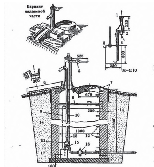
Рис. 31. Водоразборная колонка системы Черкунова: 1 — деталь эжектора и бачка; 2 — инжектор; 3 — муфта; 4 — суженный конец водопроводной трубы; 5 — противосес; 6 — лоток; 7 — штукатурка; 8 — настил из досок; 9 — воздушная трубка; 10 — вода на труба; 11 — эжектор; 12 — скобы; 13 — штанга; 14 — песок; 15 — клапан (38 мм); 16 — запорный вран; 17 — бачок
