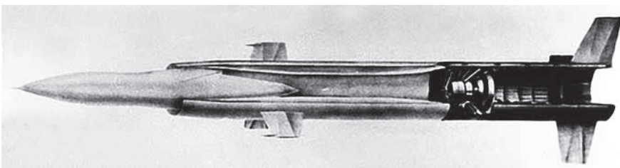
Схема ракеты комплекса «Круг» с двигателем тюменского производства
