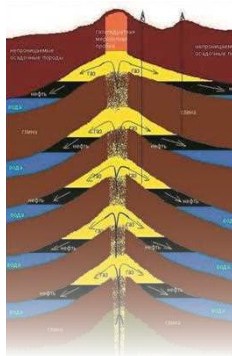
Геосолитонная модель образования восстанавливаемых залежей нефти и газа
