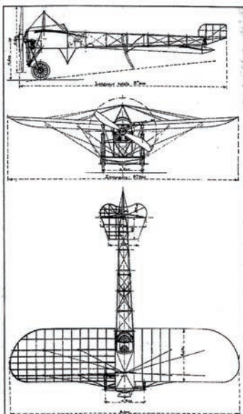
Чертёж аппарата «Блерио»
